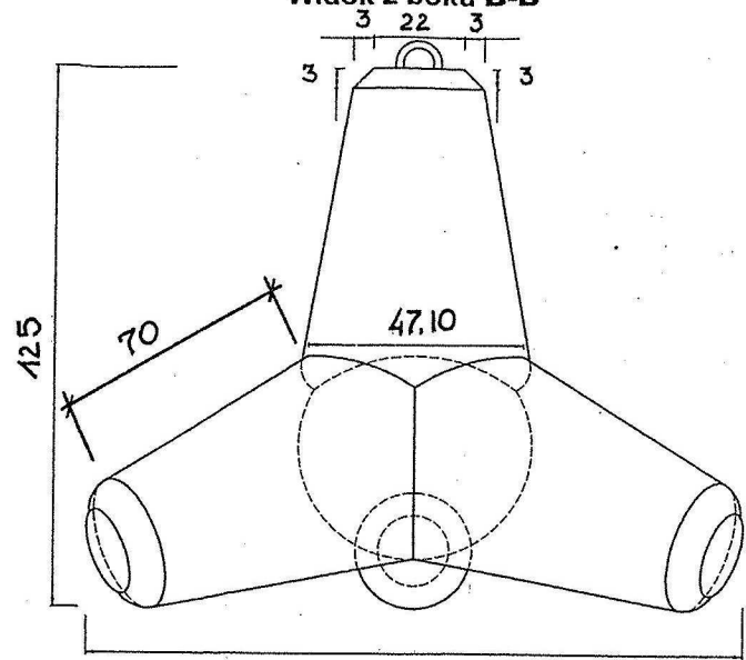
Widok z boku B-B
