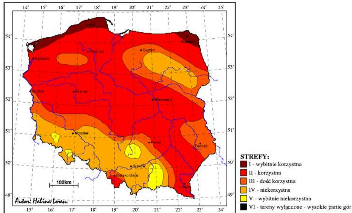
Rys. 2 Strefy energetyczne wiatru w Polsce.
