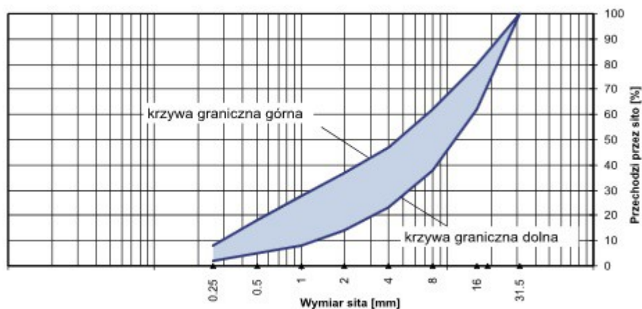
Rys. 1 Krzywe uziarnienia mieszanki betonowej
