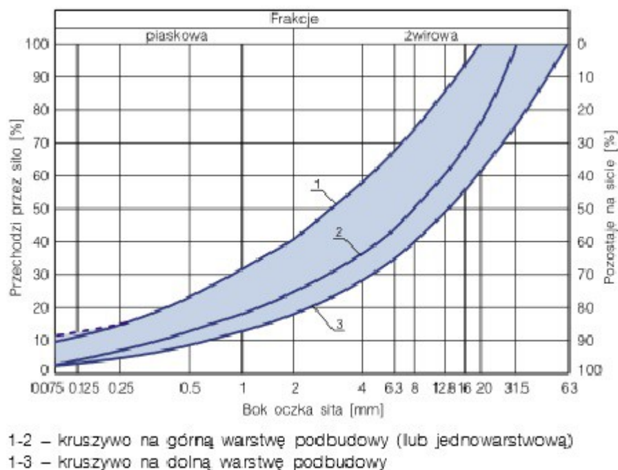
Rysunek 2 Krzywe graniczne uziarnienia wg wymagań polskich
